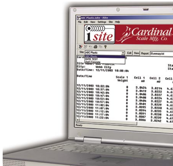
Software para monitoreo remoto de sistemas de pesaje que permite al técnico ver la operación de la balanza vía Internet.
